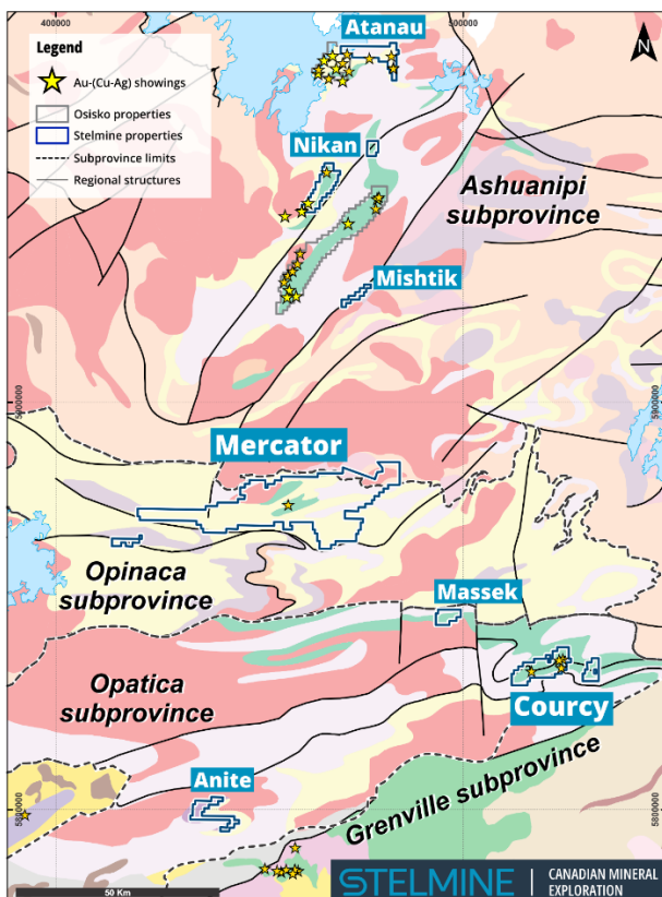
Fig. 1 : Carte géologique du district de Caniapiscou montrant la localisation des propriétés de Stelmine Canada, incluant les propriétés Atanau, Nikan et Mishtik de la sous-province d'Ashuanipi.
