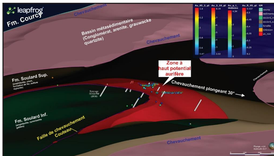
Figure 4 : Modèle 3D illustrant les divers assemblages et formations géologiques composant la propriété Courcy (zones 1 & 2) / 3D model illustrating the various rock lithologies and geological formations forming the Courcy property (zones 1 and 2).
