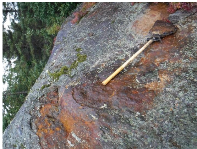
Figure 10 : Affleurement de formation de fer a grenat, magnétite et amphibole. / Iron formation outcrop rich in garnet, magnetite and amphibole.
