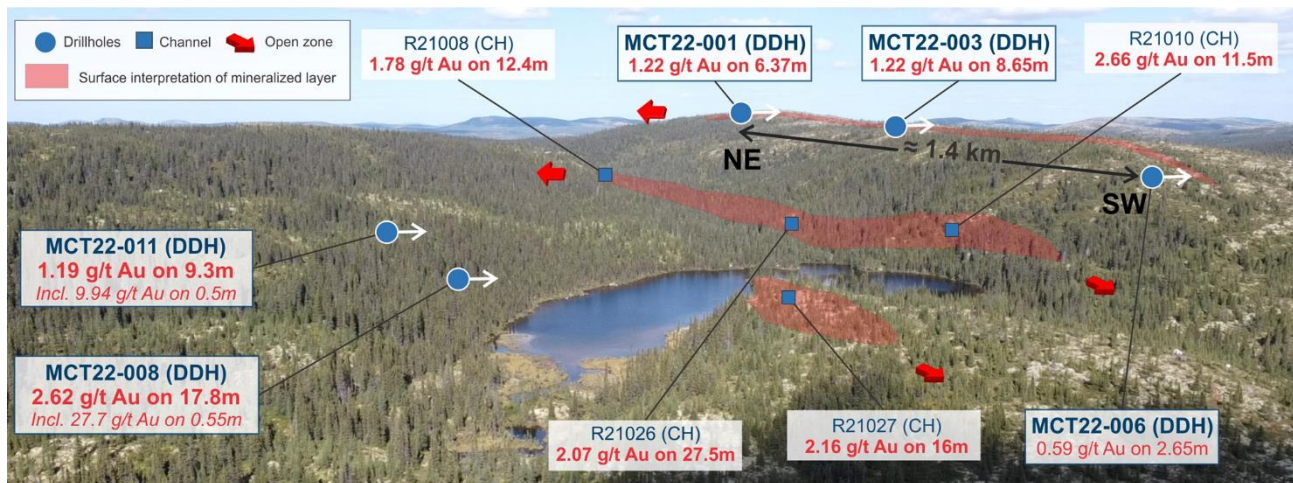
Figure 7 a) Vue vers le nord de la Zone Meridian montrant les zones minéralisées et leurs extensions probables sur le sommet d'une colline et le fond d'une vallée. / A Northeastern oblique view of a portion of the Meridian Zone showing 3 sub-parallel gold-mineralized zones on a hill crest and in a valley floor with their possible extensions,
