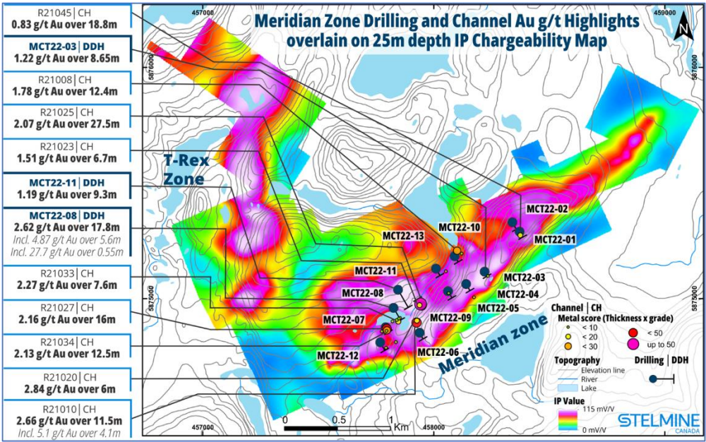
Figure 6. Carte géophysique de la Zone Meridian montrant la localisation et les teneurs aurifères d'échantillons en rainurage choisis. / Geophysical map of the Meridian Zone showing the location and gold assay values of selected channel samples.
