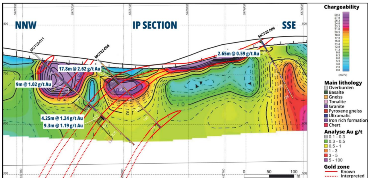
Figure 7. b) Section PP révélant la minéralisation aurifère englobée par des données de haute chargeabilité / IP Inverted section indicating most of the gold mineralization is spatially associated with high chargeability envelopes,
