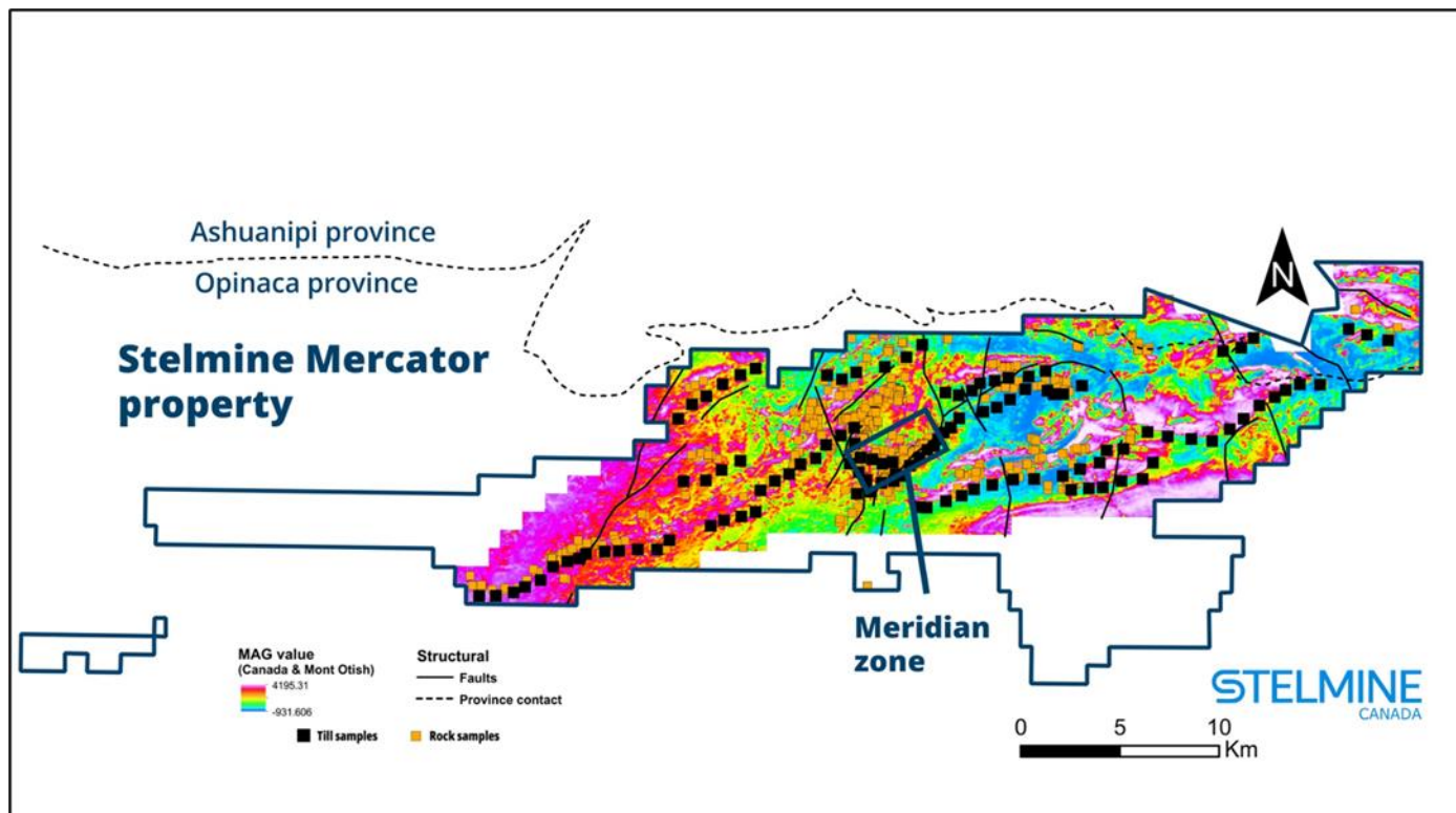
Figure. 5. Carte contour du levé hélicoptère MAG de la propriété Mercator. La localisation de la Zone Meridian et des échantillons de roche et de till à date est reportée sur la carte. / Heliborne MAG survey contour map of the Mercator property. The location of the Meridian Zone and till and rock samples to date is shown on the map.
